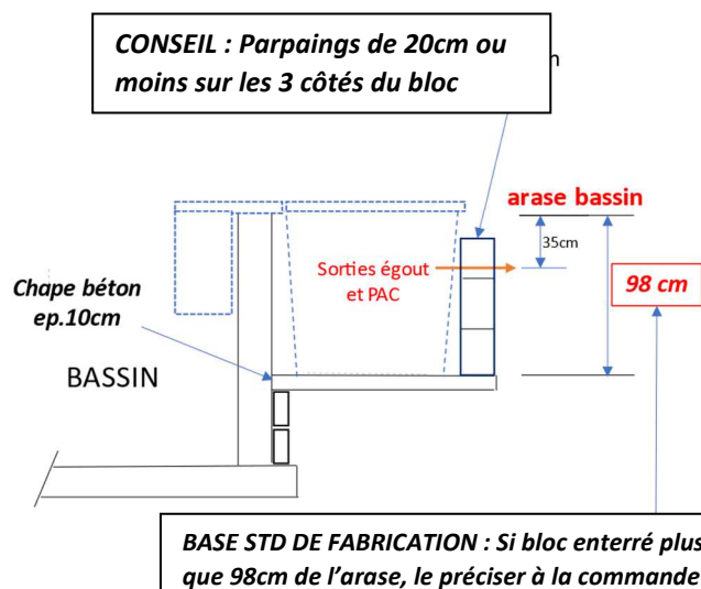
Fig.2: Vue en coupe
