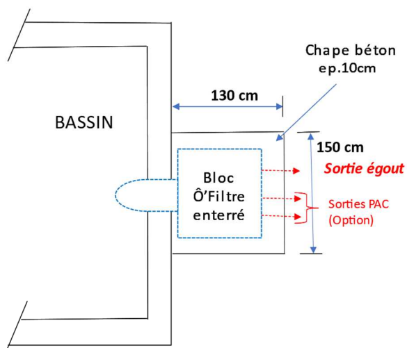
Fig.1: Vue de dessus
