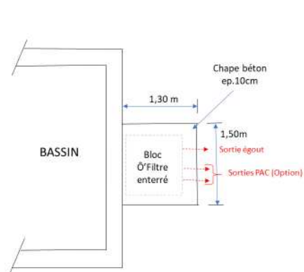
Fig.1: Vue de dessus
