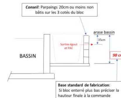
Fig.2: Vue en coupe
